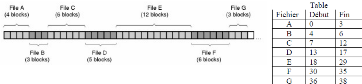
Allocation contiguë d'espace disque pour 7 fichiers
