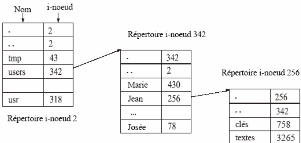
cas d'UNIX (14 octets)
