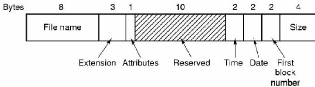
cas de MS-DOS (32 octets)
